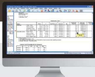
SPSS Version 24
