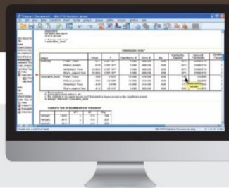
SPSS Version 24
