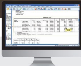
SPSS Version 24
